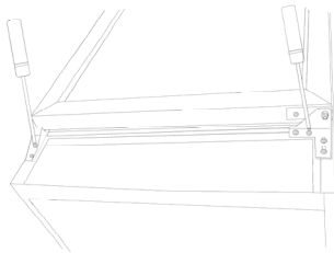
2. Remova a dobradiça superior e o acessório de suporte.
