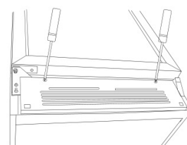
12. Riposizionare il pannello inferiore.
