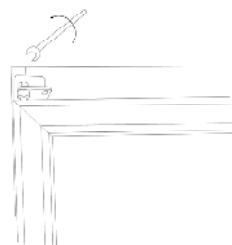
8. Den Stift vom oberen Scharnier spannen.
