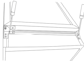
11. Kiinnitä alasarana vastakkaiselle puolelle.
