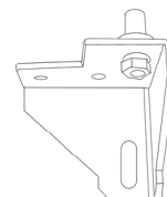
6. Den Scharnierstift in der anderen Seite montieren, aber nicht zuspanssen.
