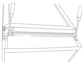
12. Montera det nedre gångjärnet på den motsatta sidan.
