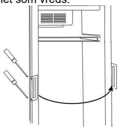
14. Flytta handtaget till den motsatta gångjärnssidan.
