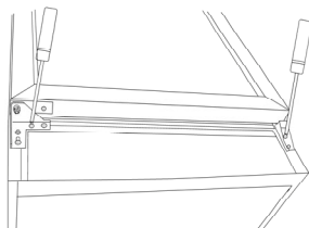
11. Monteer het onderscharnier op de tegenoverliggende kant.
