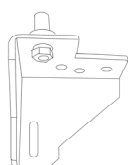
7. Podnieść drzwi na miejsce w górnym zawiasie.
