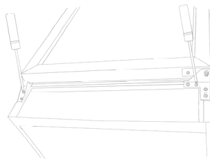
2. Retire la bisagra inferior y el accesorio de sujeción.
