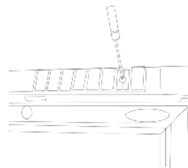
3. Retire el panel y la marquesina superiores.
