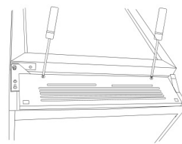
12. Ponovno namestite spodnjo ploščo.
