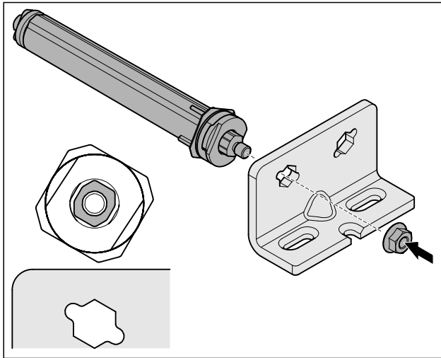
Fig. 21 Linksanschlag
