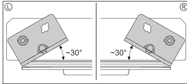
Fig. 37 Tür von unten
