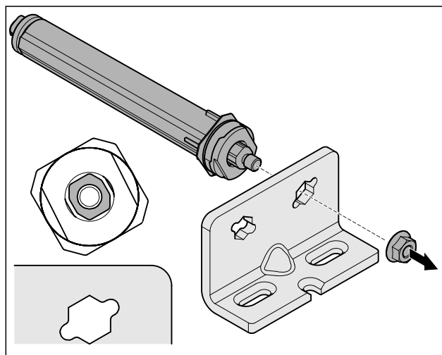
Fig. 19 Rechtsanschlag
